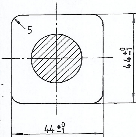
Snitt A - A
